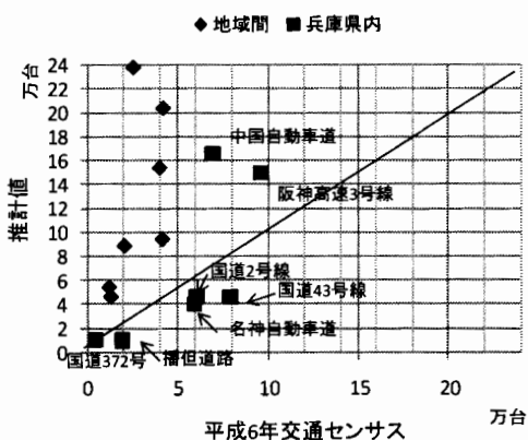
図-8 推計値と交通センサスとの比較結果 (上下両方向の交通台数の合計)
