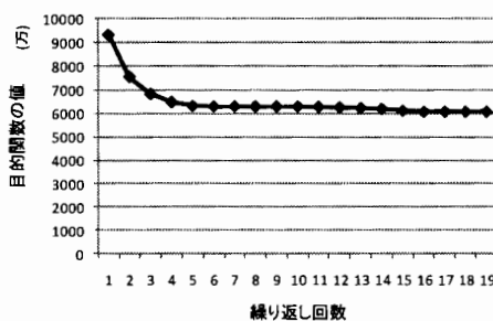
図-9 目的関数の収束の状況
