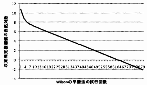
図-5 Wilsonの平衡法による収束結果(キャリブレーション終了時)
