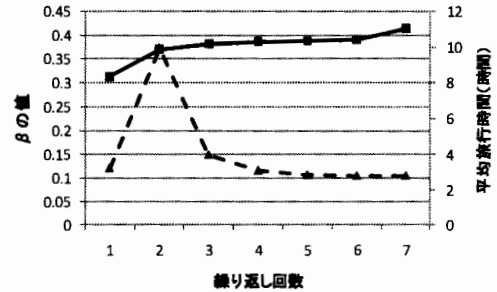
図-4 平均旅行時間の収束状況
