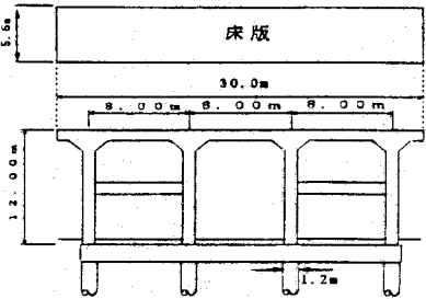
図-1 一般図
