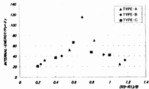
図-4 エネルギー吸収量と (R_3-R_1)/B の関係
