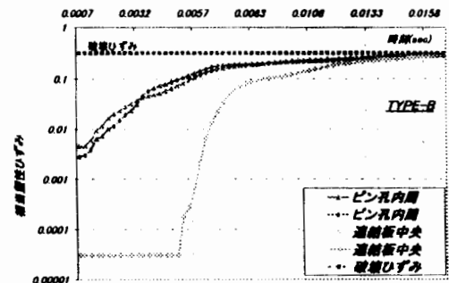
図-3 TYPE-B 相当塑性ひずみの様子
