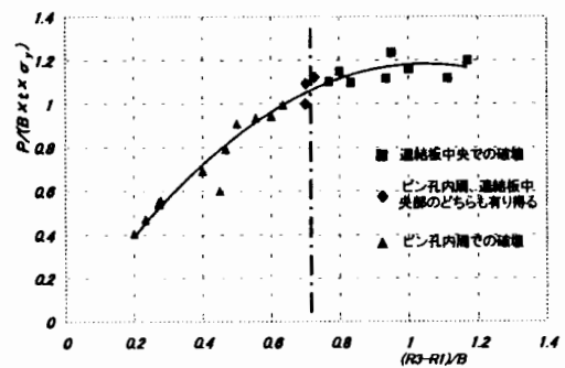
図-5 耐荷力と (R_3-R_1)/B の関係
